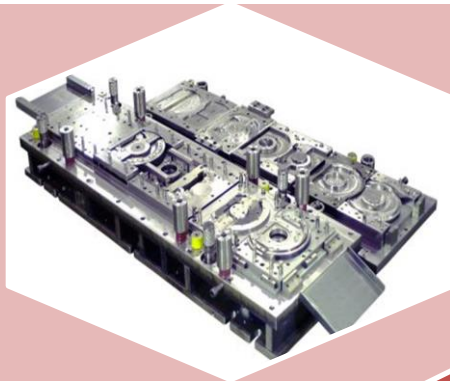
ダイカスト 用の金型
